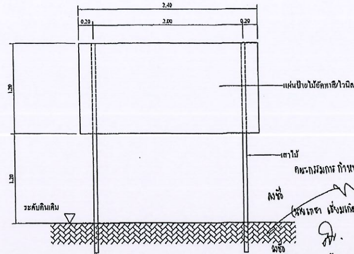
แสดงรายละเอียดโครงสร้างป้าย
