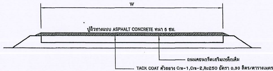
รูปตัดตามขวางโครงสร้างทาง not to scale
