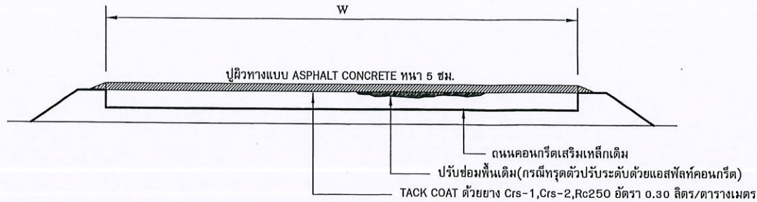
รูปตัดตามขวางโครงสร้างทาง
