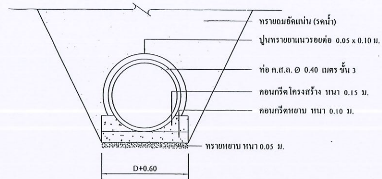
รูปตัดตามขวางท่อ มาตราส่วน 1:25
