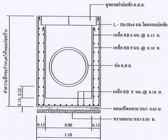
รูปตัด บ่อพัก ค.ส.ล.
