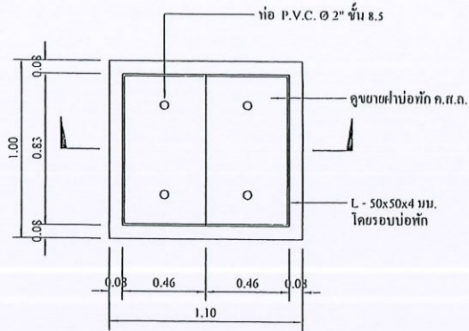
รูปแปลน บ่อพัก ค.ส.ล.ขนาด 1.00x1.10 ม. มาตราส่วน 1:25
