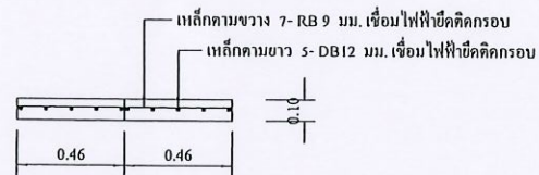
ขยาย ฝาบ่อพัก ค.ส.ล.
