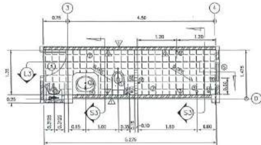
แบบสถาปัตย์ WC3 มาตราส่วน 1 : 50
