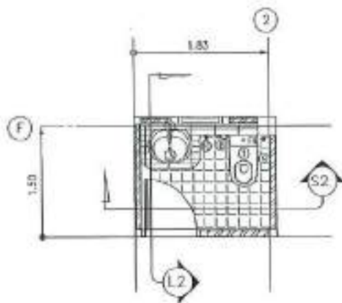
แบบแปลน WC2 มาตราส่วน 1 : 50
