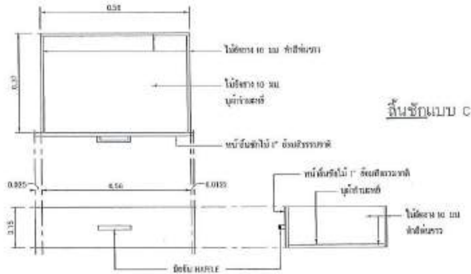
แบบขยายคู่เก็บของ (D4) มาตราส่วน 1 : 10
