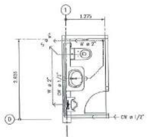
แบบสุขา WC1 มาตราส่วน 1 : 50
