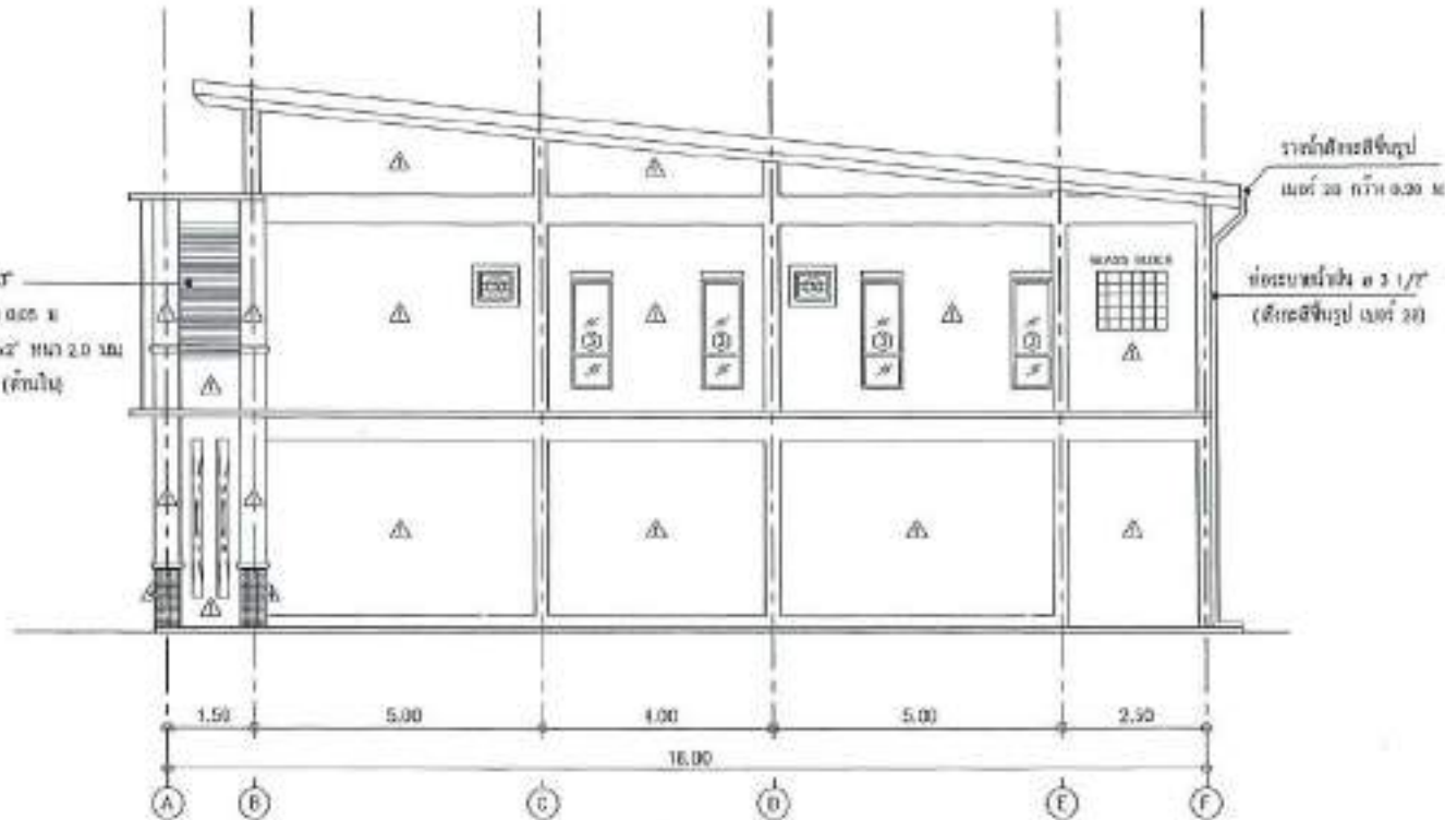
รูปด้าน 4 1/100 1 : 100
