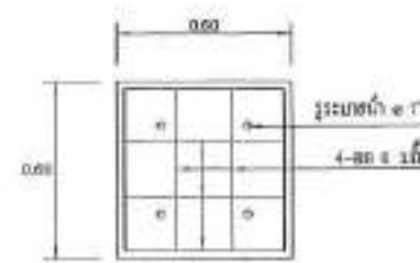
แปลนฝาบ่อพัก
