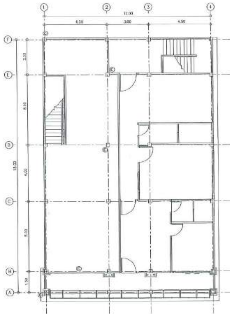
แปลนติดตั้งกล่องวงจรปิด ชั้น 2 มาตราส่วน 1 : 100
