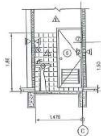
รูปตัด L4 มาตราส่วน 1 : 50
