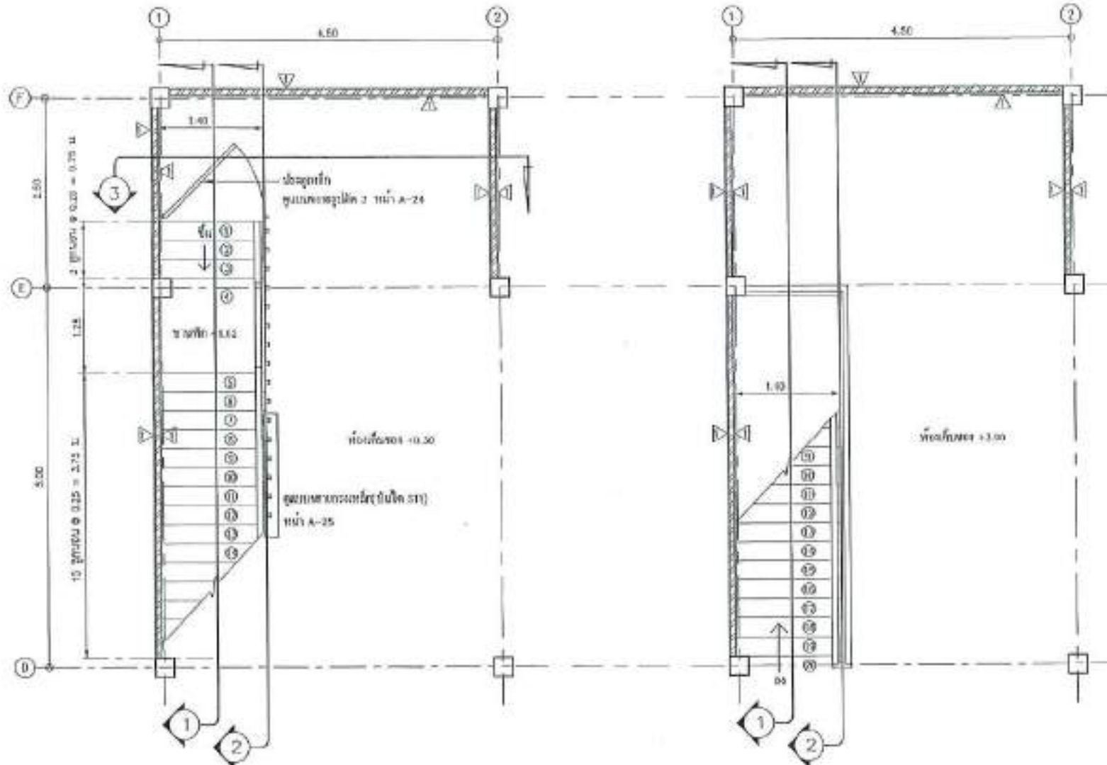
แบบแปลนบันได STI ขนาดรวม 1 : 50
