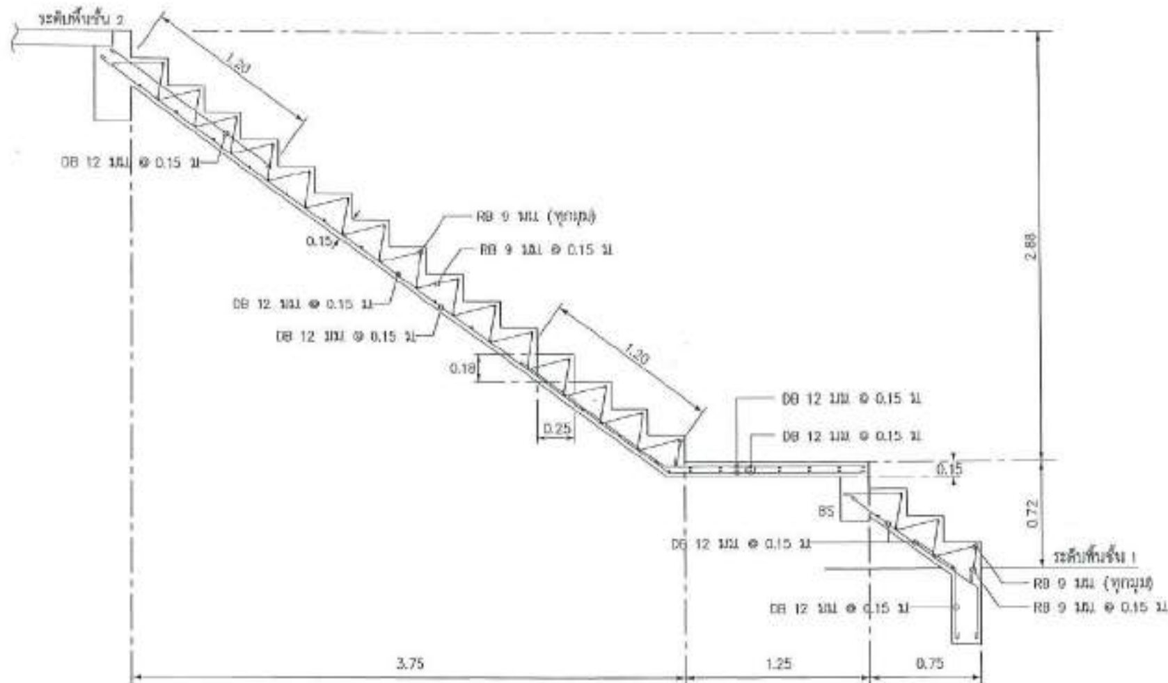
แบบขยายโครงสร้างบ้านใต้ STI มีเวลา 1.1.25
