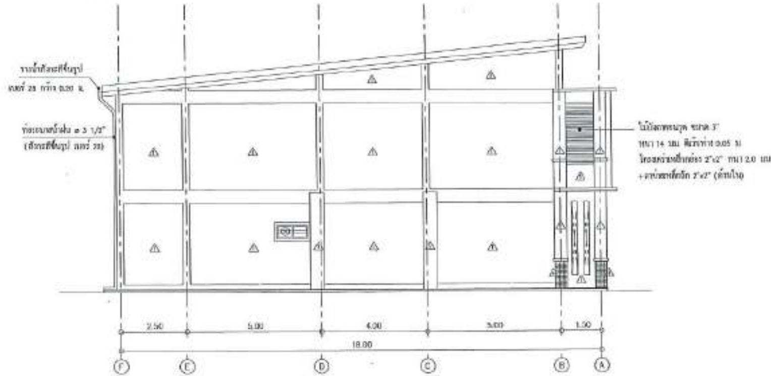
รูปด้าน 2 ขนาดจริง 1 : 100
