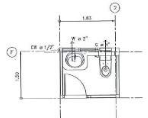
แบบสุขา WC2 มาตราส่วน 1 : 50
