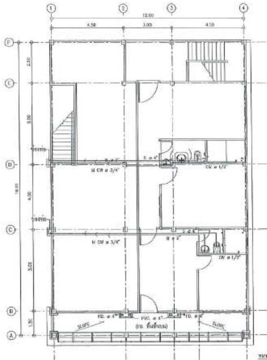
แปลนสุขาภิบาล ชั้น 2 มาตราส่วน 1 : 100
