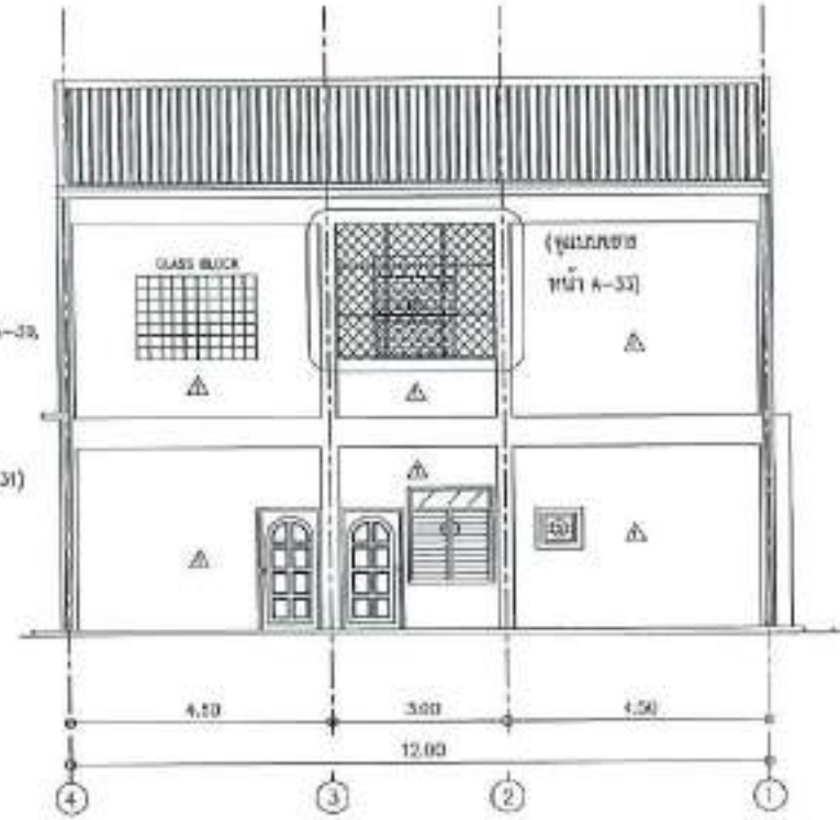
รูปด้าน 3 ขนาดส่วน 1 : 100
