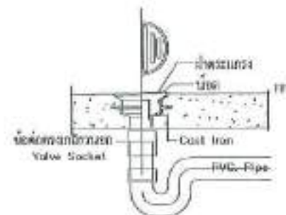
รูปแสดงการติดตั้ง Floor Drain
