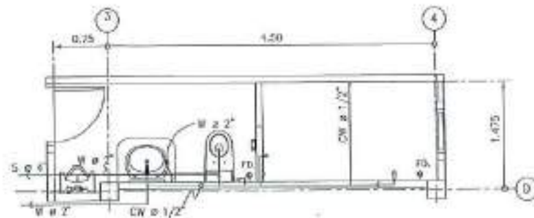
แปลนสุขาภิบาล WC2 มาตราส่วน 1 : 50
