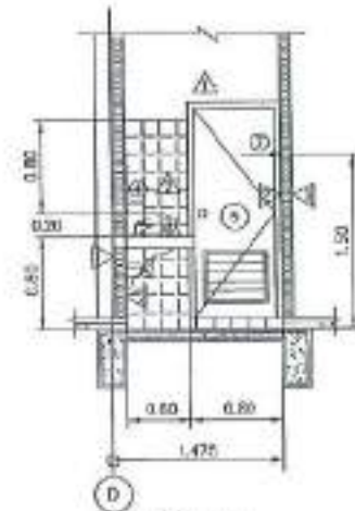
รูปตัด S3 มาตราส่วน 1 : 50
