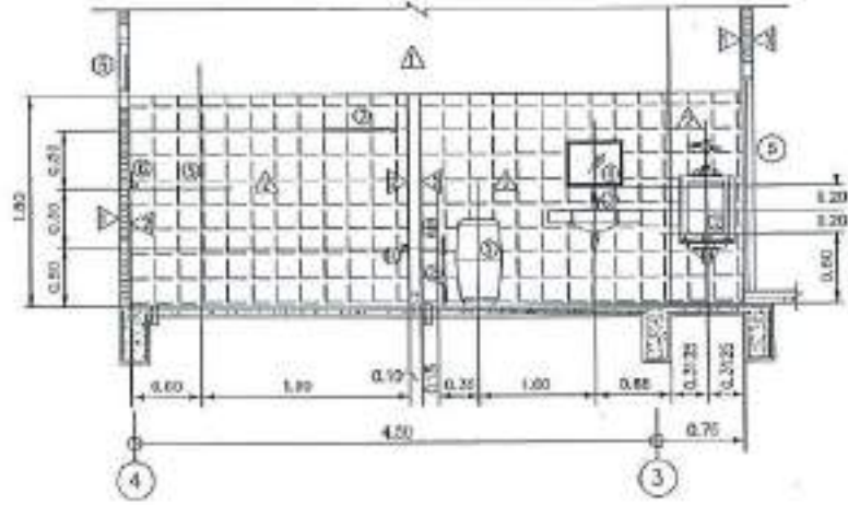
รูปตัด L3 มาตราส่วน 1 : 50
