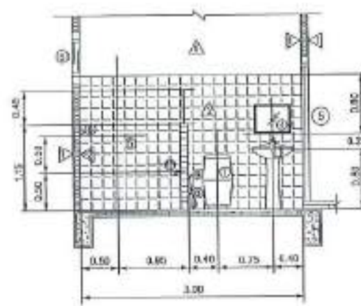
รูปตัด L4 มาตราส่วน 1 : 50
