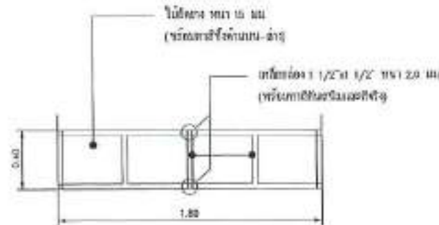
รูปด้าน G
