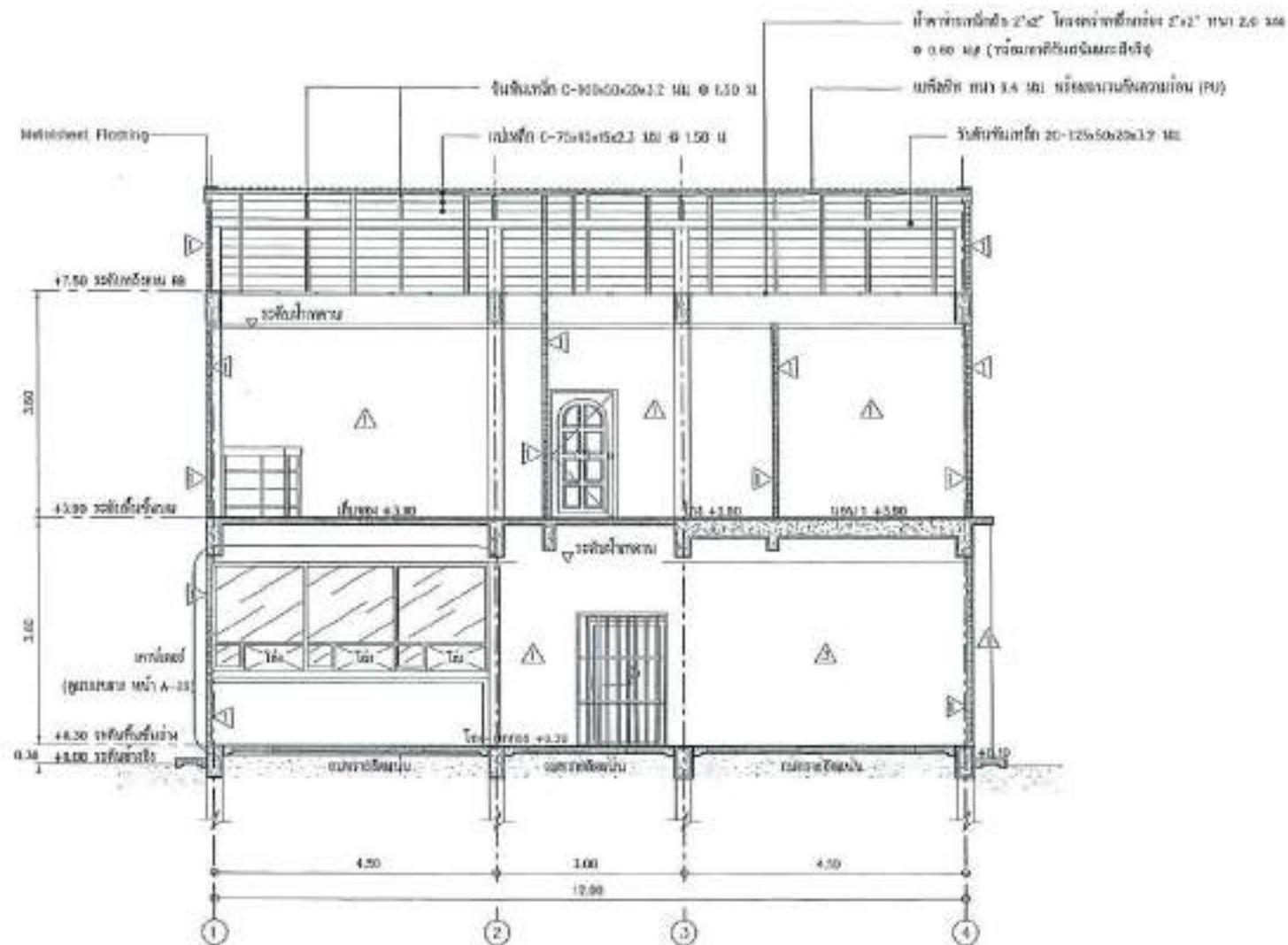
รูปตัด A มาตราส่วน 1 : 75
