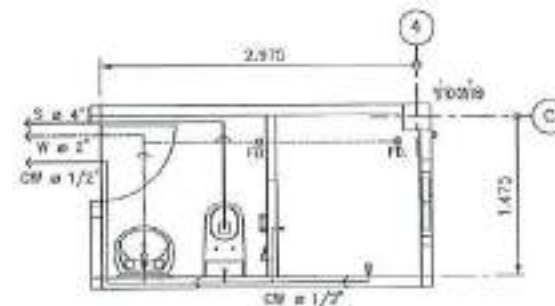
แปลนสุขาภิบาล WC3 มาตราส่วน 1 : 50
