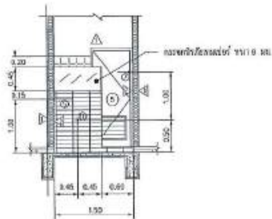
รูปตัด S4' มาตราส่วน 1 : 50
