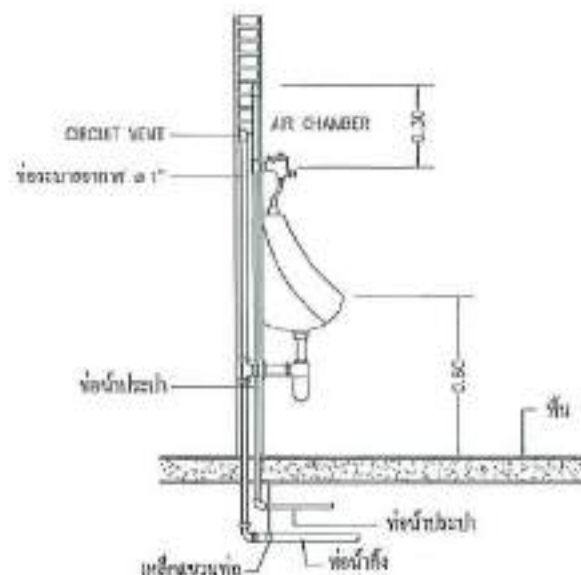
โถปัสสาวะผู้ชาย
