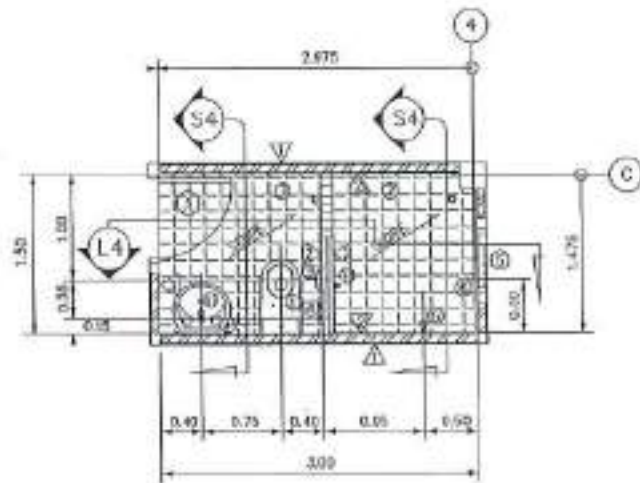
แบบร่าง WC4 มาตราส่วน 1 : 50
