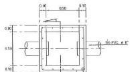
แปลนบ่อพัก
