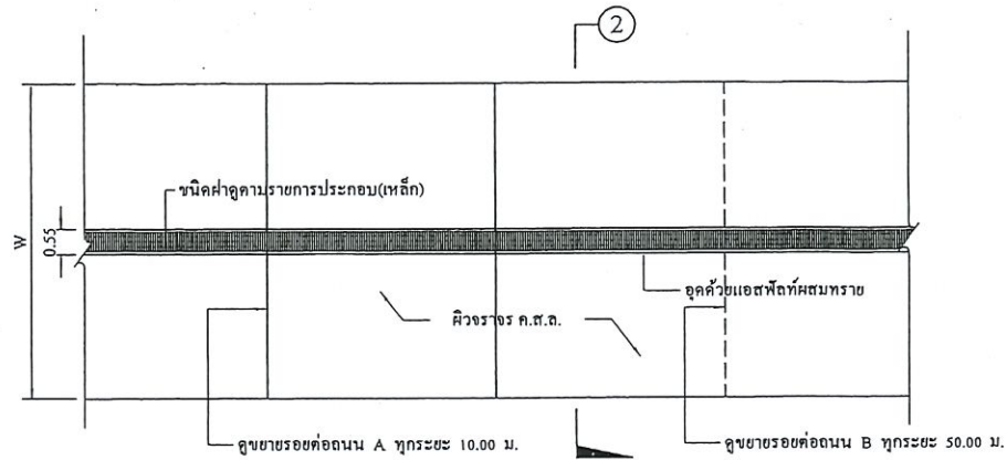
แปลนถนน ค.ส.ล.และวางระบายน้ำรูปตัวยู กรณีวางระบายน้ำอยู่กลางถนน
