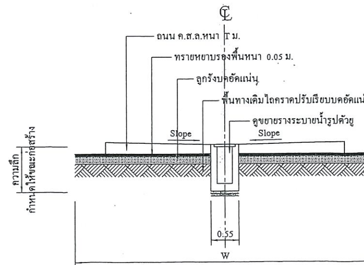
รูปตัด 2 (กรณีวางระบายน้ำอยู่กลางถนน)
