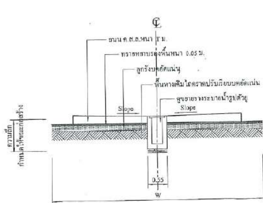
รูปตัด 2 (กรณีรางระบายน้ำอยู่กลางถนน)
