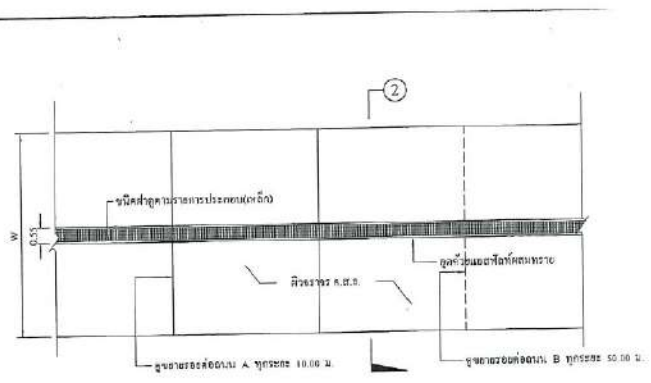
แปลนถนน ค.ส.ล.และรางระบายน้ำรูปตัววี กรณีรางระบายน้ำอยู่กลางถนน
