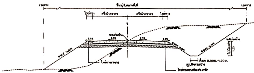
รูปตัดขวางแบบสันดินและคันดิน
