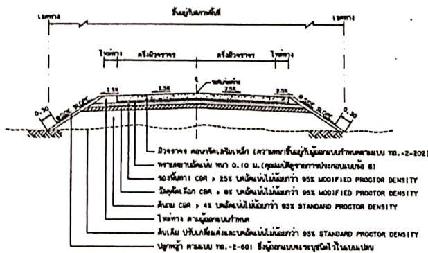
รูปตัดขวางโครงสร้างถนนลาดยางสันดินและคันดิน
