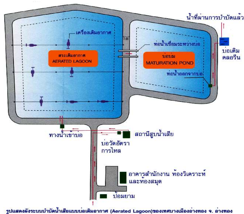
รูปที่ 5 – 3 ผังระบบบำบัดน้ำเสียแบบบ่อเติมอากาศ เทศบาลเมืองอ่างทอง
