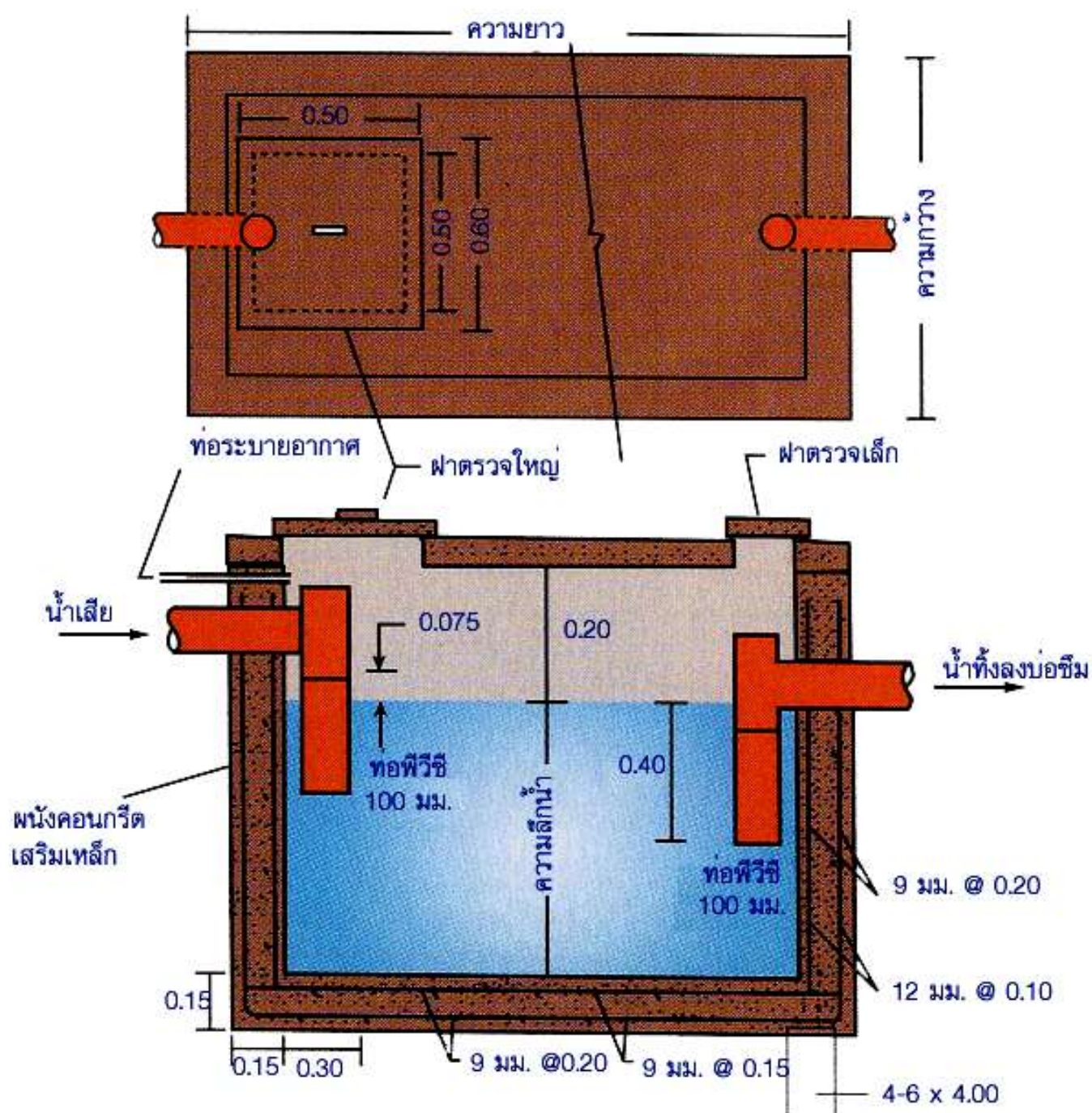
แบบมาตรฐานบ่อเกราะขนาดเล็ก
