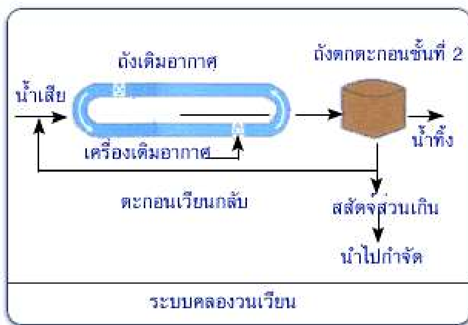
รูปที่ 5 – 6 ผังกระบวนการบำบัดน้ำเสียแบบแอคติเวเต็ดสลัดจ์แบบคลองวนเวียน
