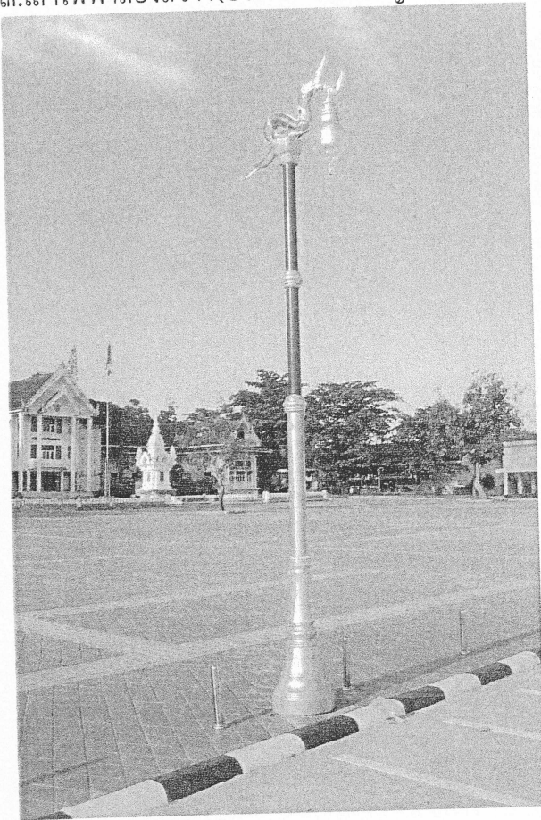
๓.เสาไฟฟ้าส่องสว่าง(ประติมากรรมพญานาค) ขนาดสูง ๓ เมตรและ ๖ เมตร
