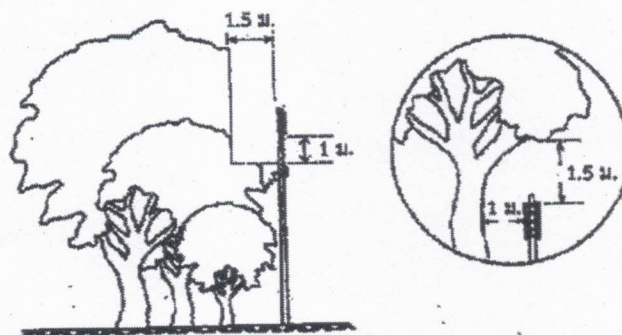
ภาพที่ 4 การตัดต้นไม้ใกล้ระบบจำหน่ายแรงต่ำ
