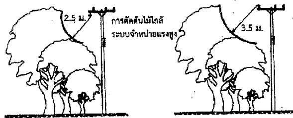
ภาพที่ 2 กรณีสายไฟฟ้าแรงสูงเป็นขั้วหม้อแปลงเบี่ยง ระยะห่างต่ำสุดหลังการตัด ทุกทิศทางไม่น้อยกว่า 3.50 เมตร
