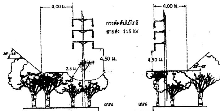
ภาพที่ 4 กรณีไม่มีระบบจำหน่ายแรงสูงได้แนวสายส่ง
