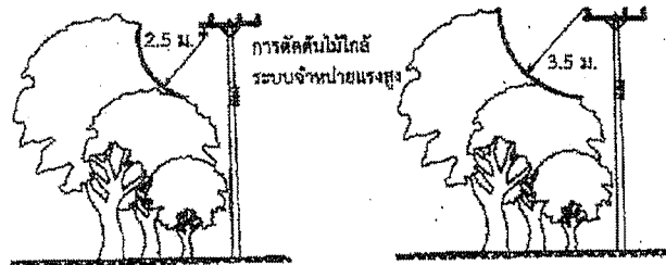
ภาพที่ 2 กรณีสายไฟฟ้าแรงสูงเป็นดุมเปลือย ระยะห่างต่ำสุดหลังการตัด ทุกทิศทางไม่น้อยกว่า 3.50 เมตร
