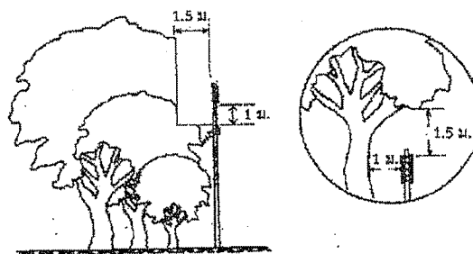
ภาพที่ 5 การตัดต้นไม้ใกล้ระบบจำหน่ายแรงต่ำ
