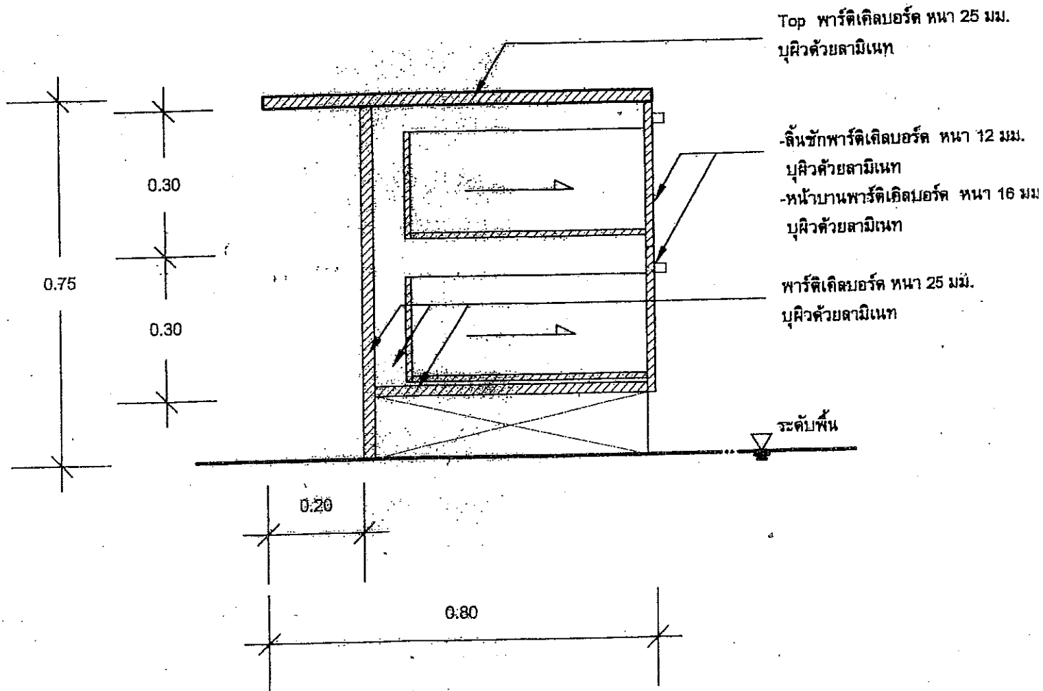
รูปตัด มาตราส่วน 1:10
