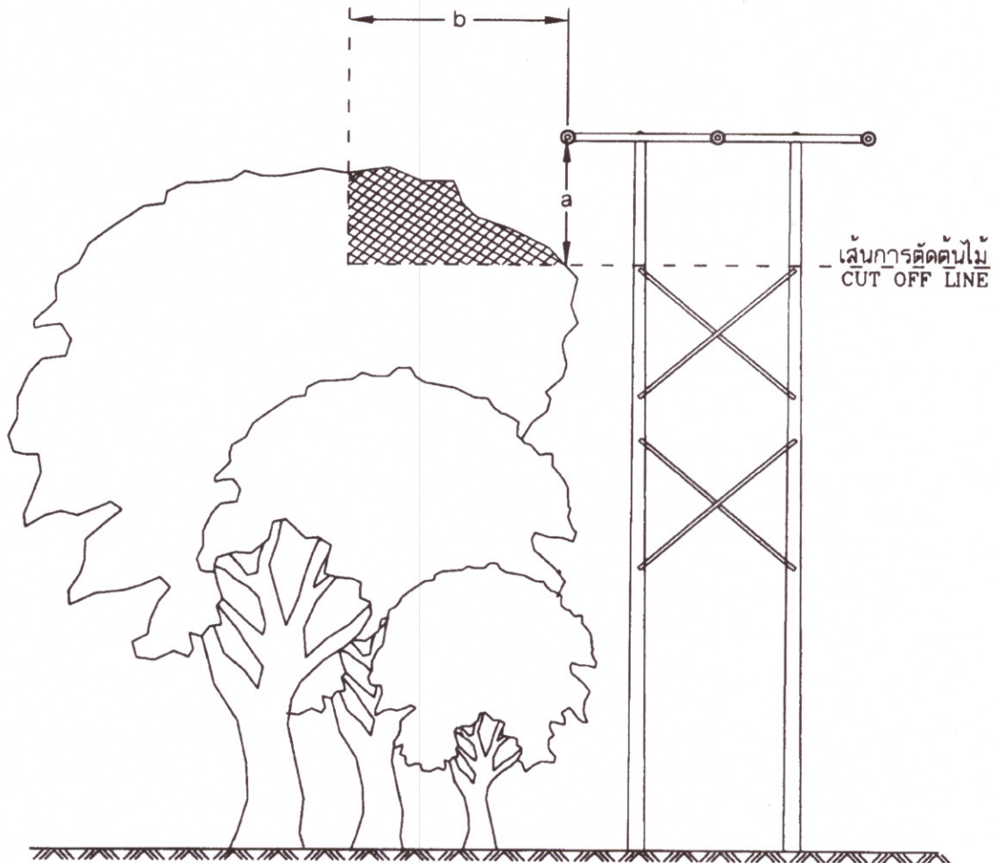
การตัดแต่งต้นไม้สำหรับสายเบลี้อยแรงสูงที่มีระยะห่างระหว่างเสาตั้งแต่ 100 เมตร ขึ้นไป TREE TRIMMING FOR H.V. BARE CONDUCTOR WITH SPANS OF 100 m AND ABOVE.
