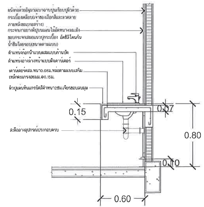
แบบขยายรูปตัดขวางเคาน์เตอร์ในห้องน้ำ
