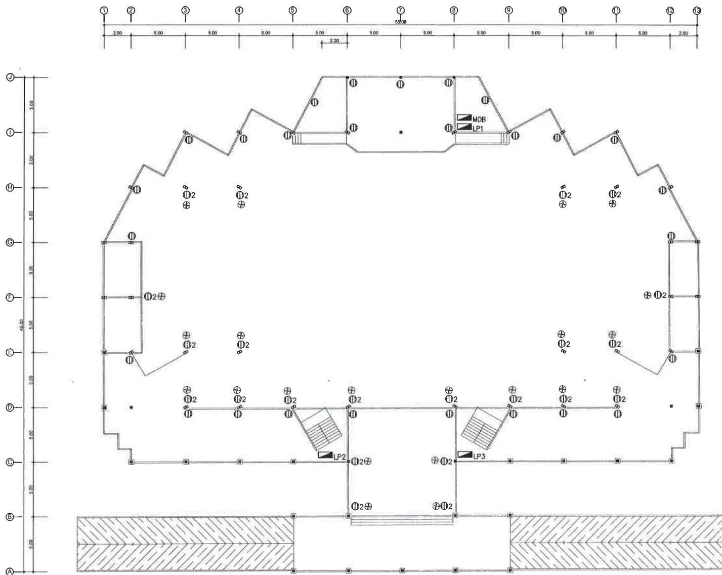
แปลนระบบไฟฟ้าชั้นบน มาตราส่วน 1 : 250
