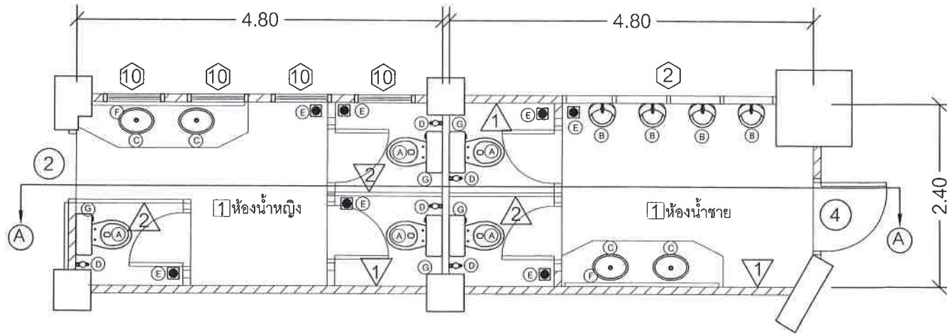
แบบแปลนห้องน้ำชั้นบน (ใหม่) ขนาดส่วน 1:50
