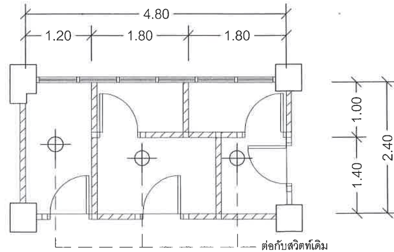
แปลนระบบไฟฟ้าห้องน้ำชั้นล่าง มาตราส่วน 1:50
