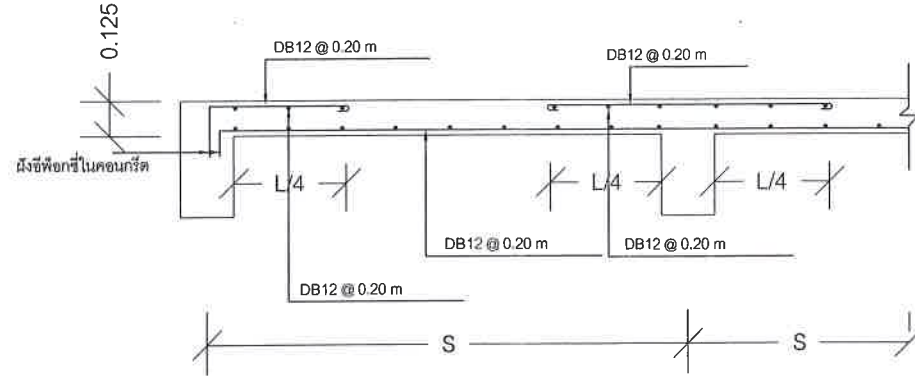
ขยายพื้น S1 มาตราส่วน NTS
