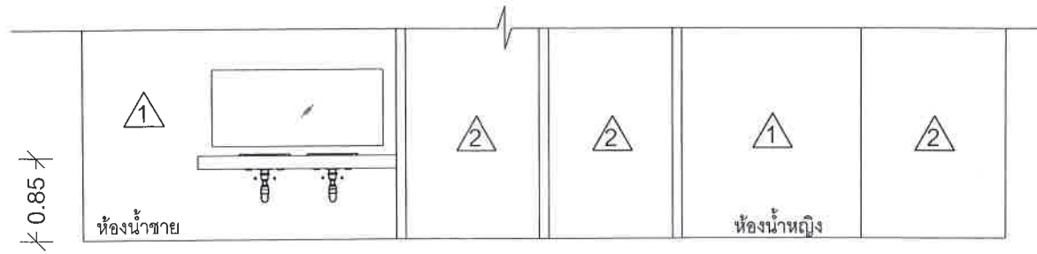
รูปตัดแนว A - A มาตราส่วน 1:50
