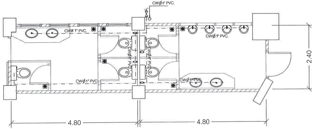
แปลนระบบน้ำ มาตราส่วน 1:50
