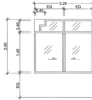
ขยายหน้าต่าง (8)
