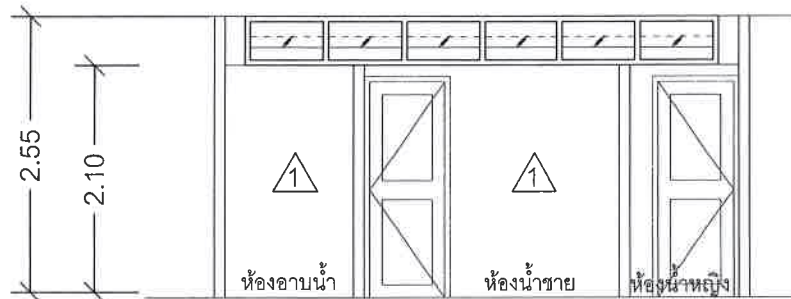
รูปตัดแนว B - B มาตราส่วน 1:50
