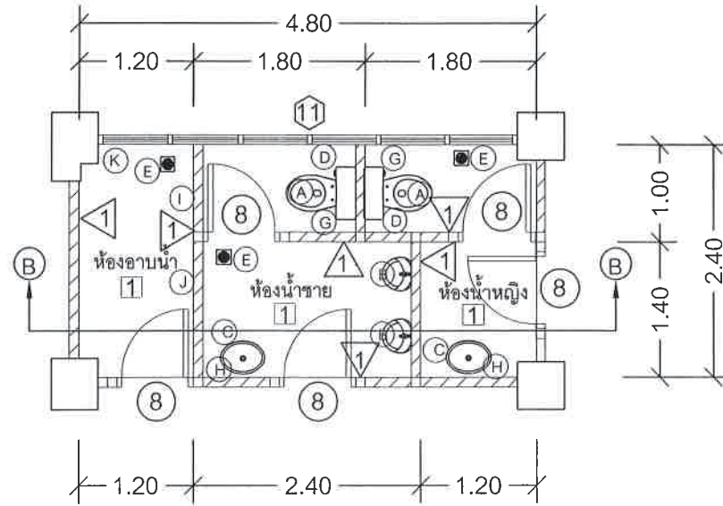
แบบแปลนห้องน้ำชั้นล่าง มาตราส่วน 1:50
