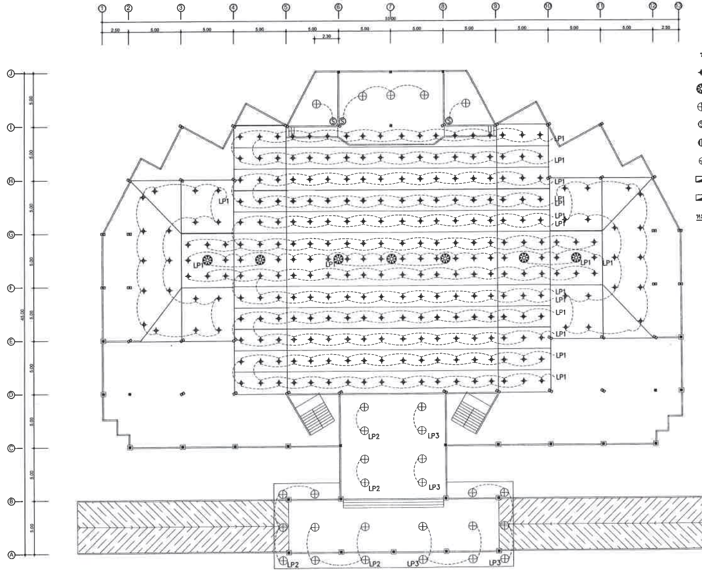
แปลนระบบไฟฟ้าแสงสว่างชั้นบน มาตราส่วน 1 : 250
