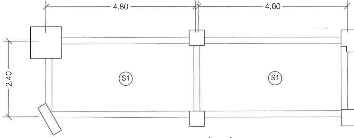
แปลนโครงสร้างพื้นห้องน้ำ มาตราส่วน 1:50
