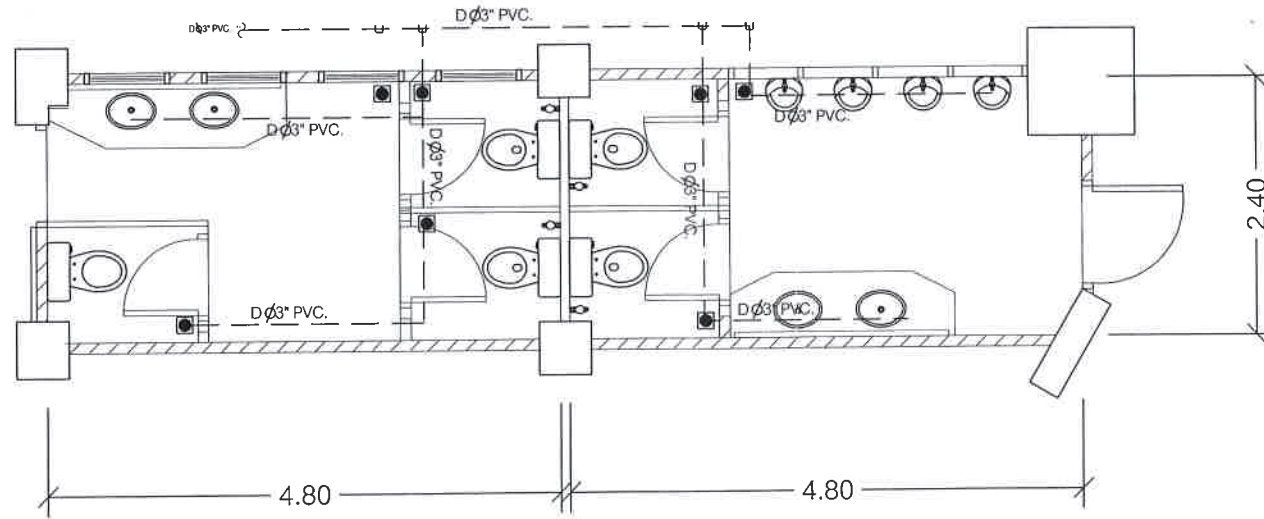
แปลนระบบน้ำเสีย มาตราส่วน 1:50
