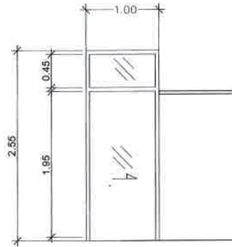
ขยายประตู ②
