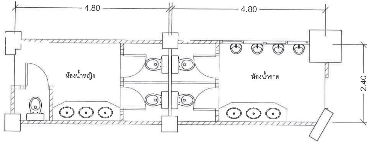
แบบแปลนห้องน้ำชั้นบน (เดิม) ขนาดส่วน 1:50
