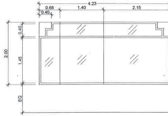
ขยายหน้าต่าง (9)
