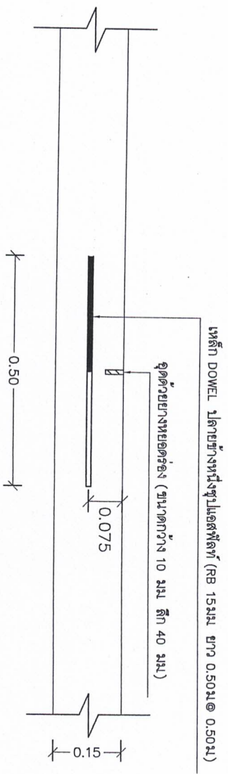
รอยต่อเพื่อการหดตัว (CONTRACTION JOINT) มาตราส่วน 1 : 10
