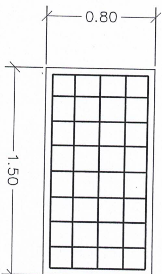
แบบขยาย F1 มาตราส่วน 1:20
