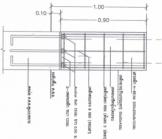
แบบขยาย คอนกรีตเสริมเหล็ก มาตราส่วน NTS
