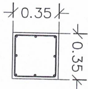
แบบขยาย C1 มาตราส่วน 1:20
